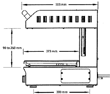
側視圖
