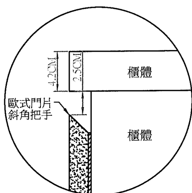
歐式門片細部圖
