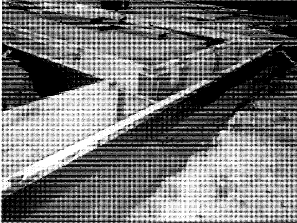
排水管線配置
