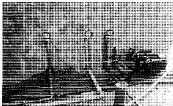
管線壓力測試
