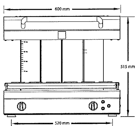
正視圖
